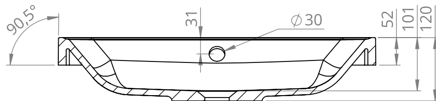
PRZEKRÓJ G-G SKALA 1 : 7
